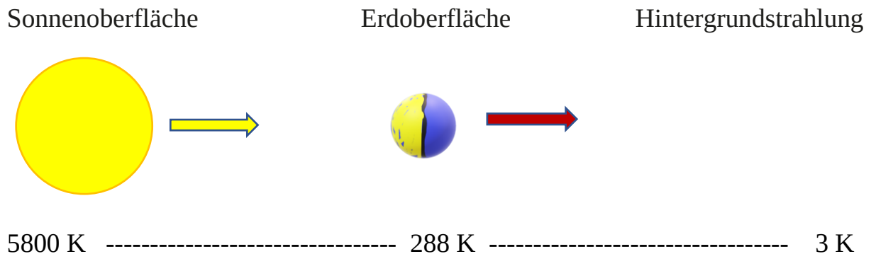
Abb. 2. Energieflüsse und Temperaturverhältnisse des Systems Sonne/Erde/All.
